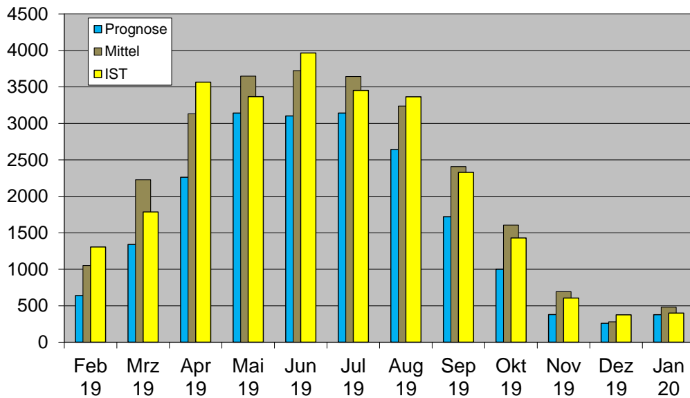
Energie [kWh] 12-Monats-Vergleich Krippe + Bürgerhalle
