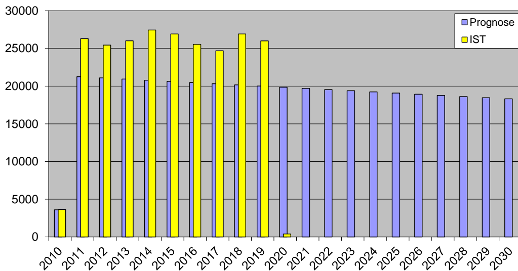
kWh Prognose- und IST, Energie pro Jahr, Krippe + Bürgerhalle
